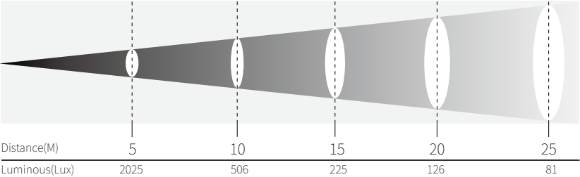
Beam Angle: 52°
